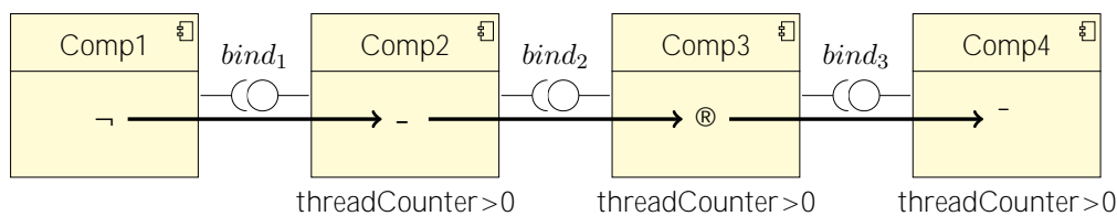
Figura 4.7: O fluxo de execução num componente.
