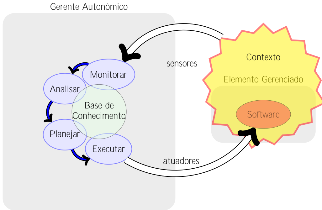
Figura 2.4: Atividades do ciclo de decisão MAPE-K (adaptado de KEPHART e CHESS (2003)).
