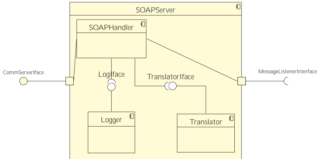
Figura 5.6: Diagrama do componente SOAPServer.
