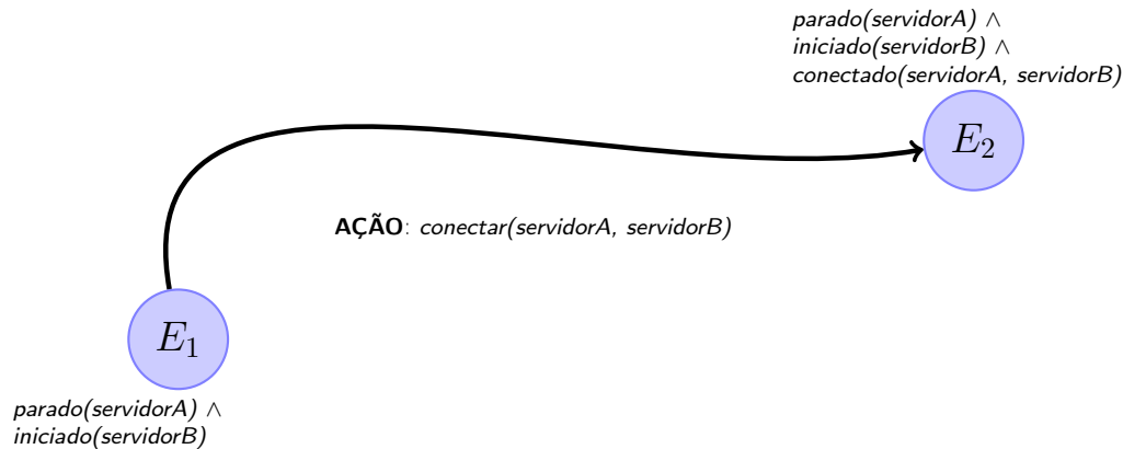
Figura 2.1: Transição entre configurações.
