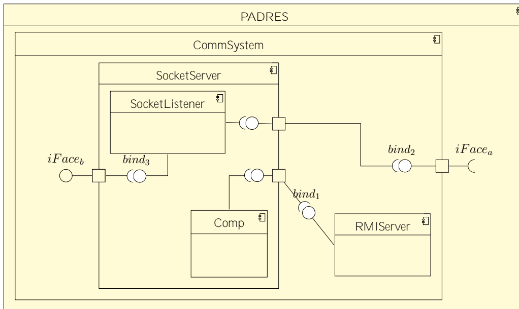
Figura 4.3: Tipos de enlaces de interfaces requeridas pelo componente SocketServer.
