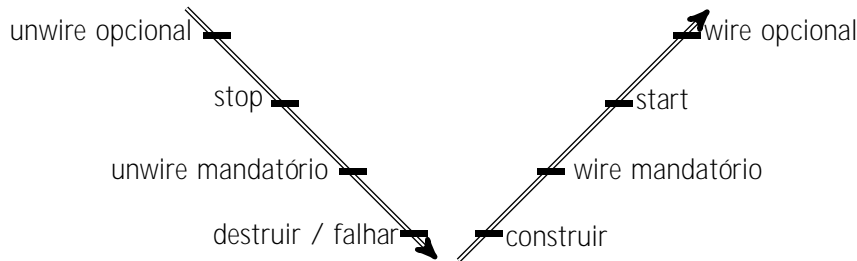
Figura 3.7: A ordem entre as ações de reconfiguração nas fases “para baixo” e “para cima”.
