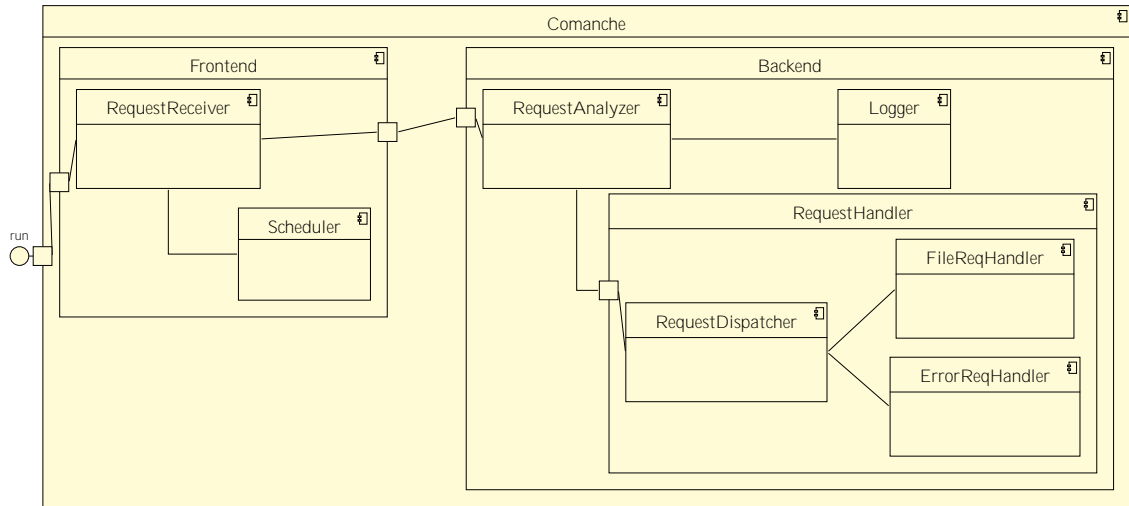
Figura 5.1: Diagrama de Componentes do Servidor Comanche.
