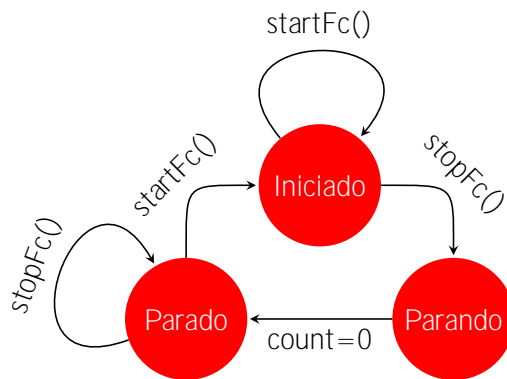
Figura 4.6: Ciclo de vida de um componente em Julia.
