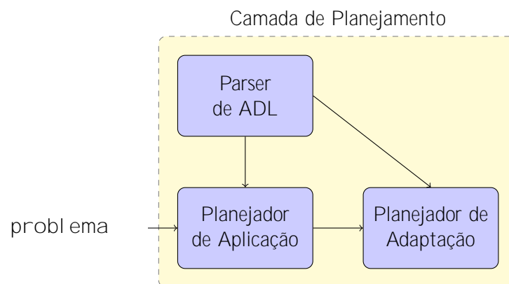
Figura 3.3: Camada de Planejamento - adaptado de TAJALLI et al. (2010)
