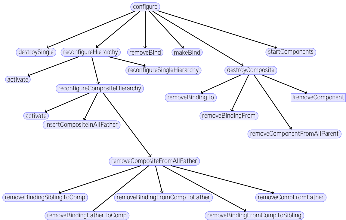
Figura 4.18: Um grafo ilustrando a ordem entre alguns métodos de decomposição pertencentes ao domínio de planeamento.
