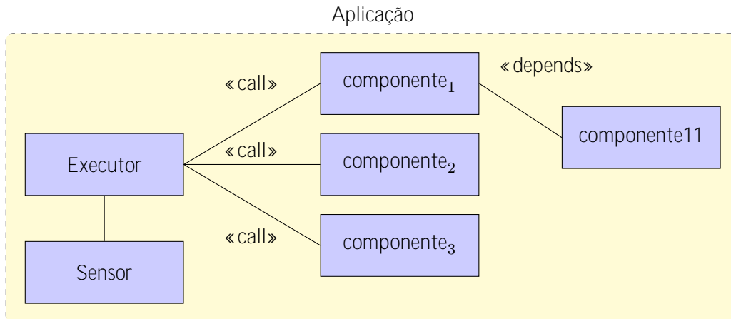
Figura 3.4: Arquitetura da aplicação a ser executada no robô - adaptado de TAJALI et al. (2010)
