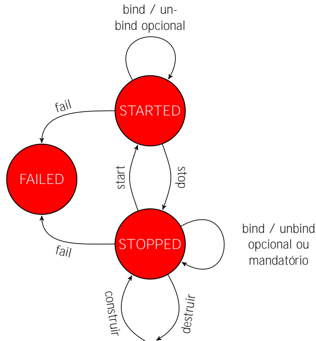
Figura 3.5: Um grafo ilustrando a gramática de reconfiguração.
