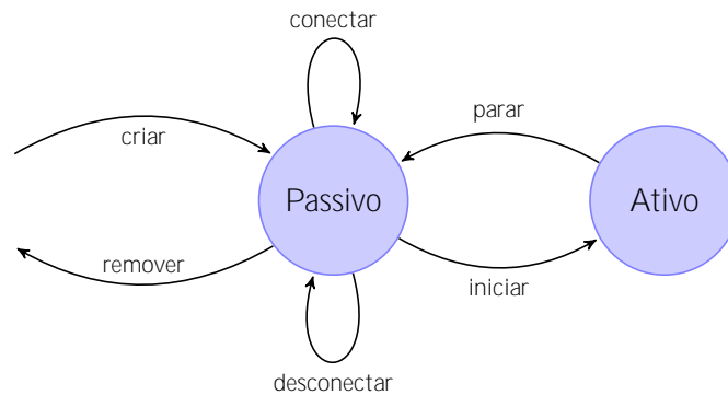
Figura 2.8: As transições entre os estados do ciclo de vida de um componente, segundo KRAMER e MAGEE (1990).
