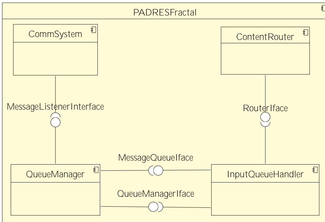
Figura 4.11: Diagrama de componentes de uma configuração.
