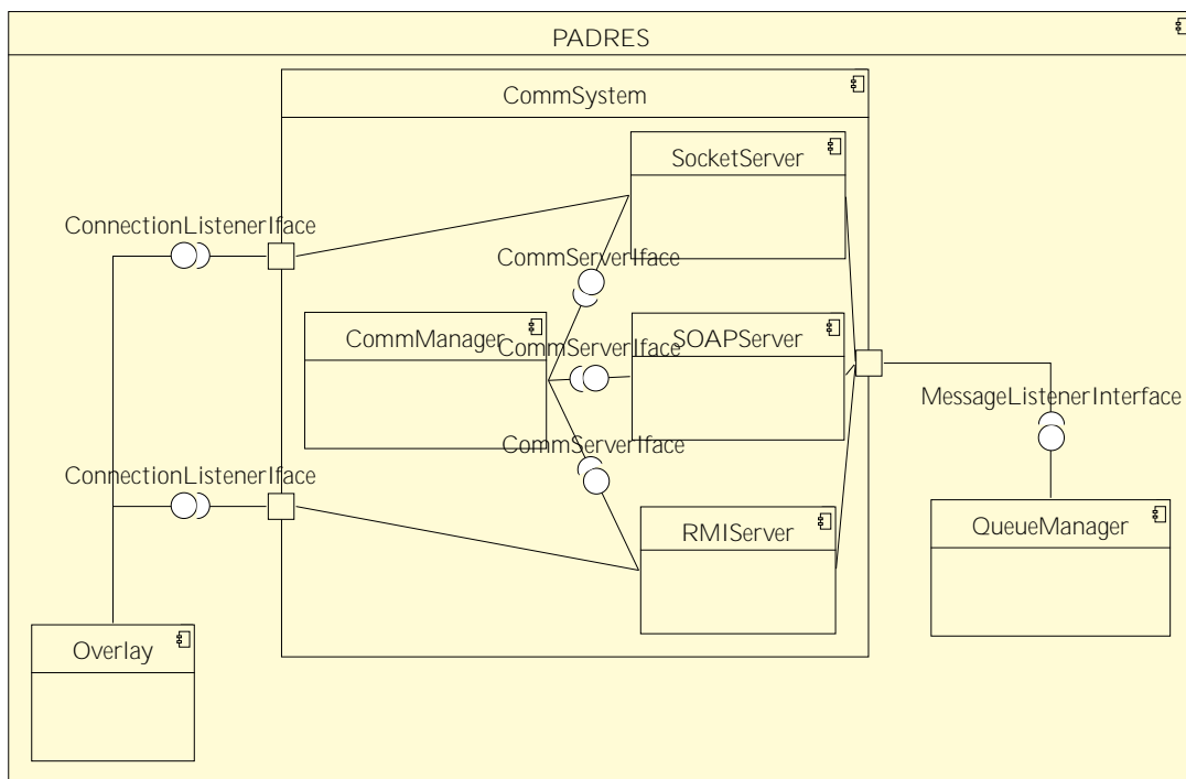
Figura 5.5: Trecho da Configuração Objetivo do Componente Composto CommSystem.
