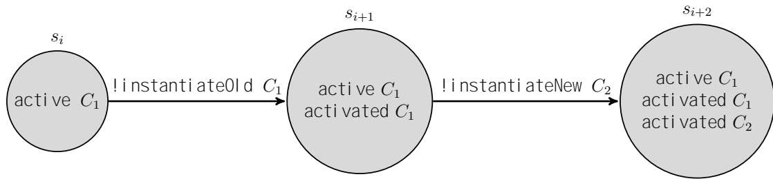
Figura 4.12: Um diagrama de transição de estados.
