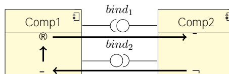
Figura 4.8: Dependência circular.
