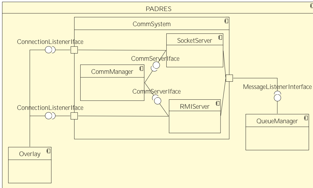
Figura 5.3: Diagrama do Componente Composto CommSystem.
