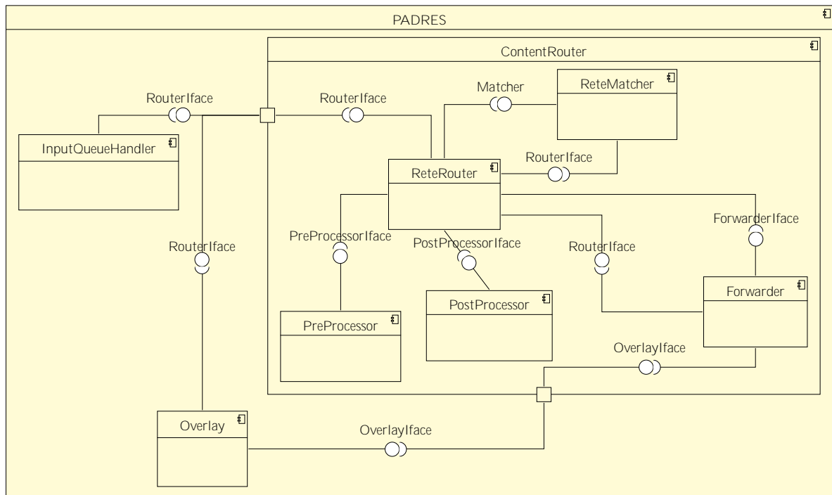
Figura 5.4: Diagrama do Componente Composto ContentRouter.
