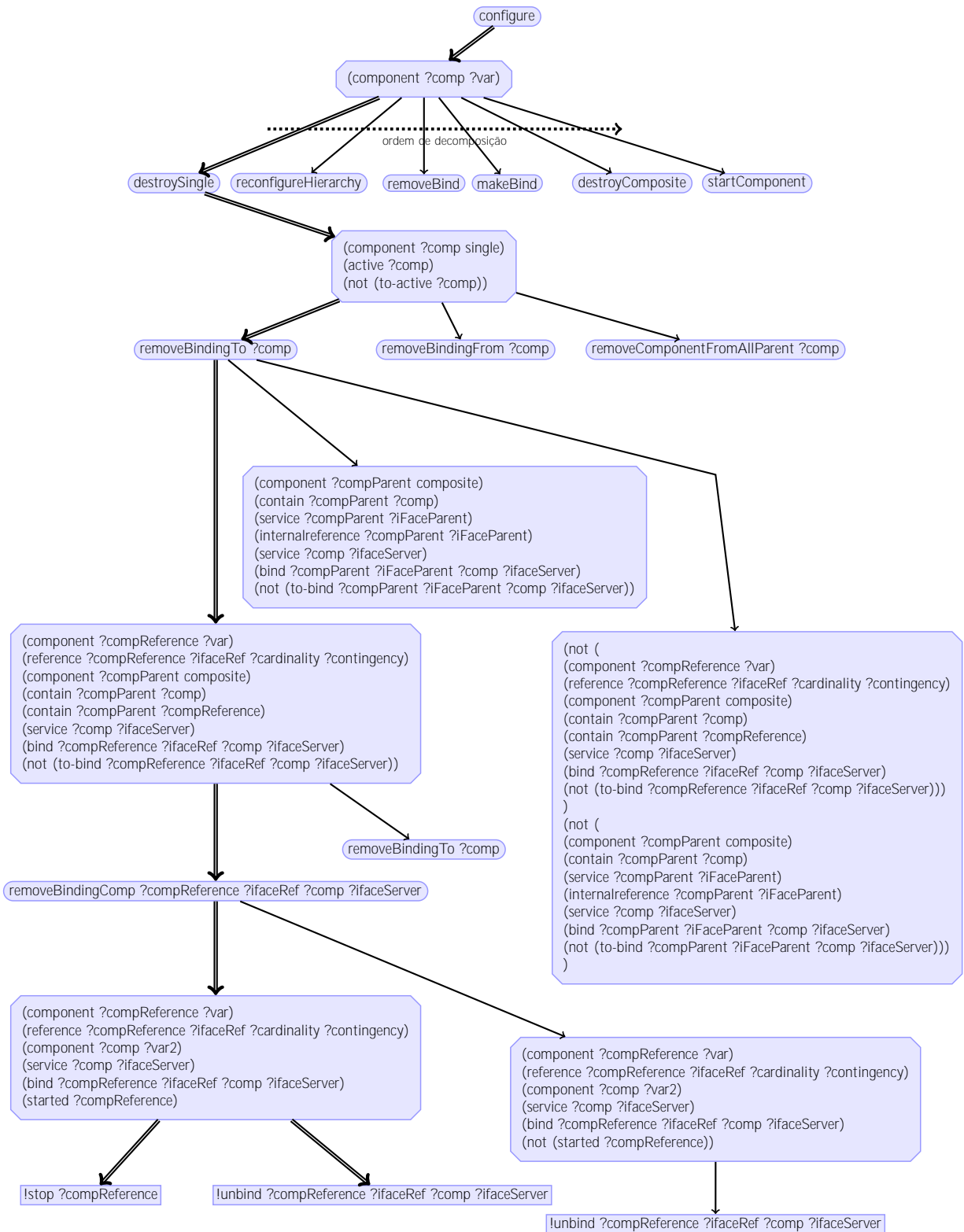
Figura 4.16: Uma representação gráfica da rede de tarefas dos métodos: configure , destroySingle , removeBindingTo e removeBindingComp .
